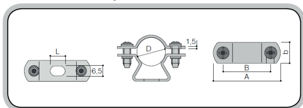
disegno dimensionale / reference details
